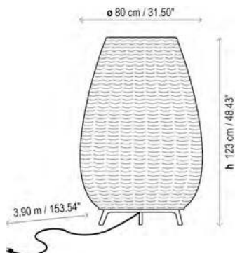
Amphora 02 IP-66
